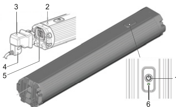
Illustration 36 : Vue d'ensemble de la batterie SHIMANO BT-E8036
