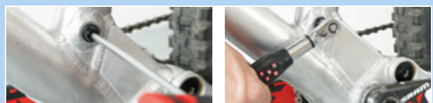
Illustration 207 : Fixer l'axe Postpin
