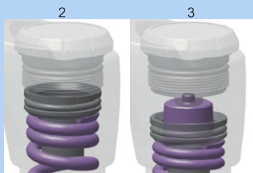
Illustration 99 : Serrer et desserrer l'anneau de réglage de la prétension
