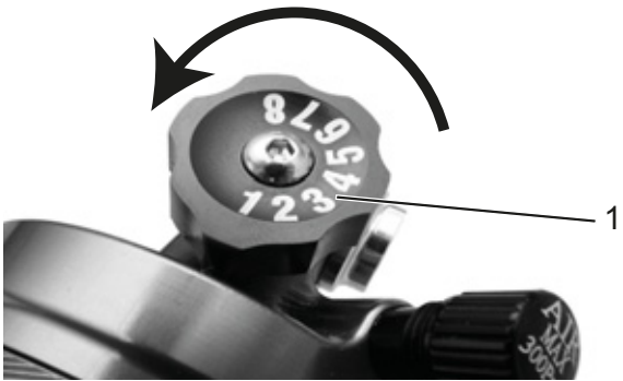
Illustration 260 : Réglage de la compression Suntour (1) sur l'amortisseur arrière
