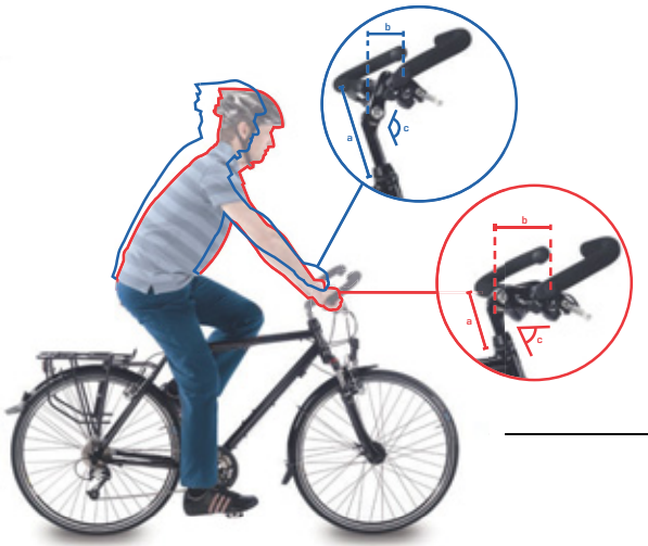
Illustration 86 : Position sur vélo de ville (en bleu) et sur vélo tout chemin (en rouge) avec modification de l'angle
