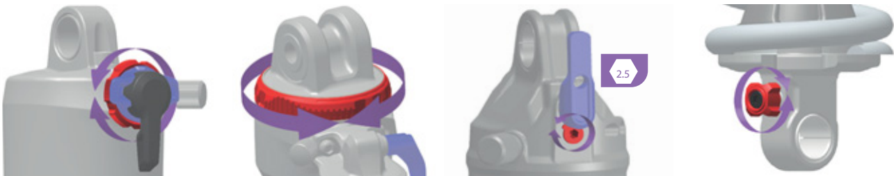
Illustration 266 : La position et la forme du dispositif de réglage de la détente (rouge) dépendent du modèle
