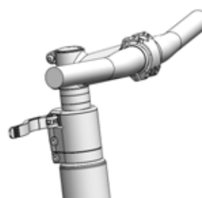
Illustration 157 : All Up avec levier de serrage de la potence ouvert
