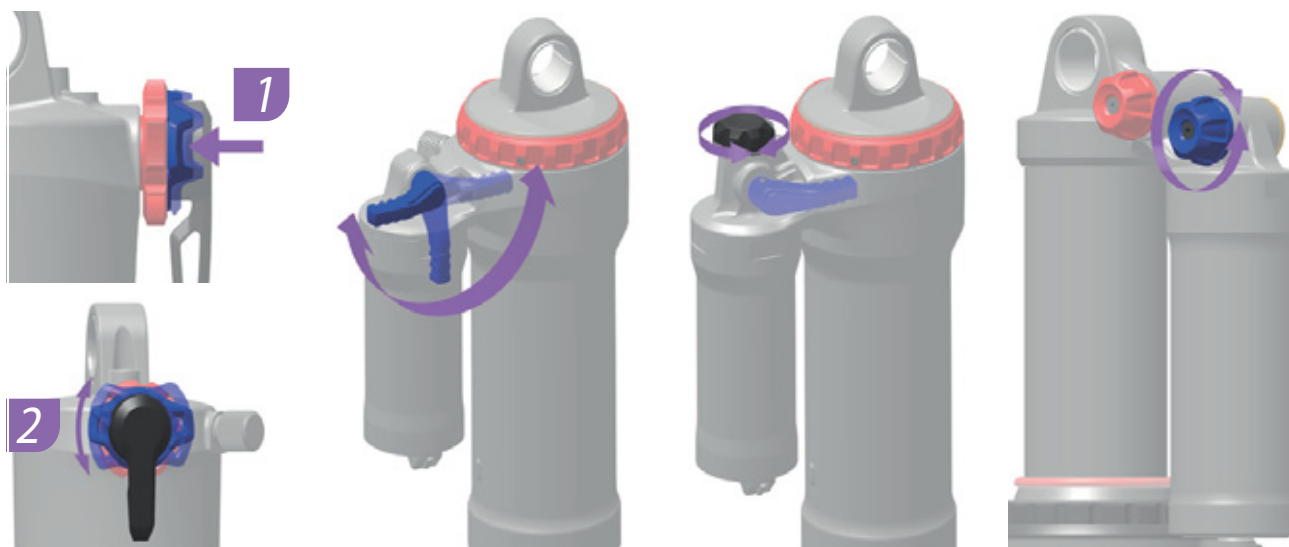
Illustration 119 : La position et la forme du dispositif de réglage de la compression (bleu) dépendent du modèle
