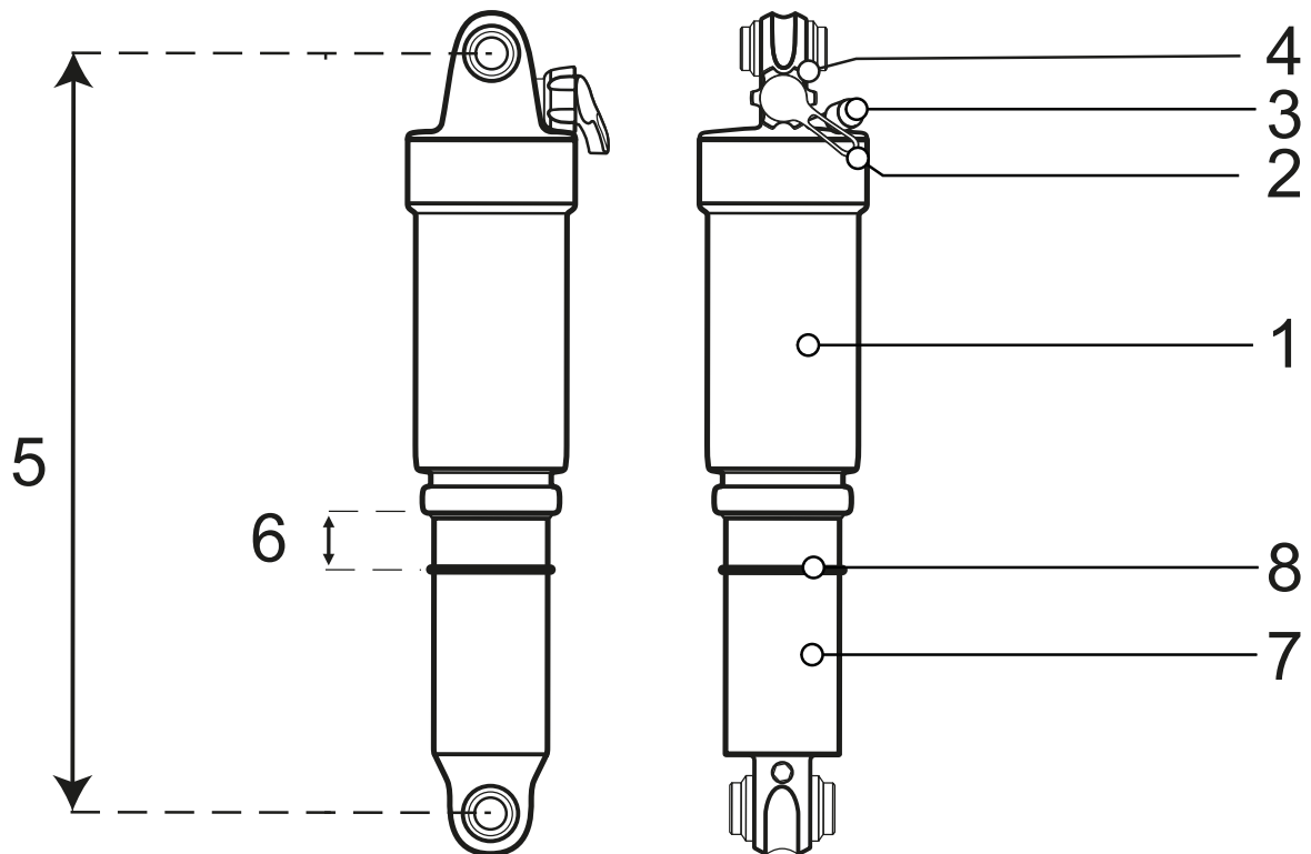
Illustration 20 : Exemple d'un amortisseur arrière Suntour
